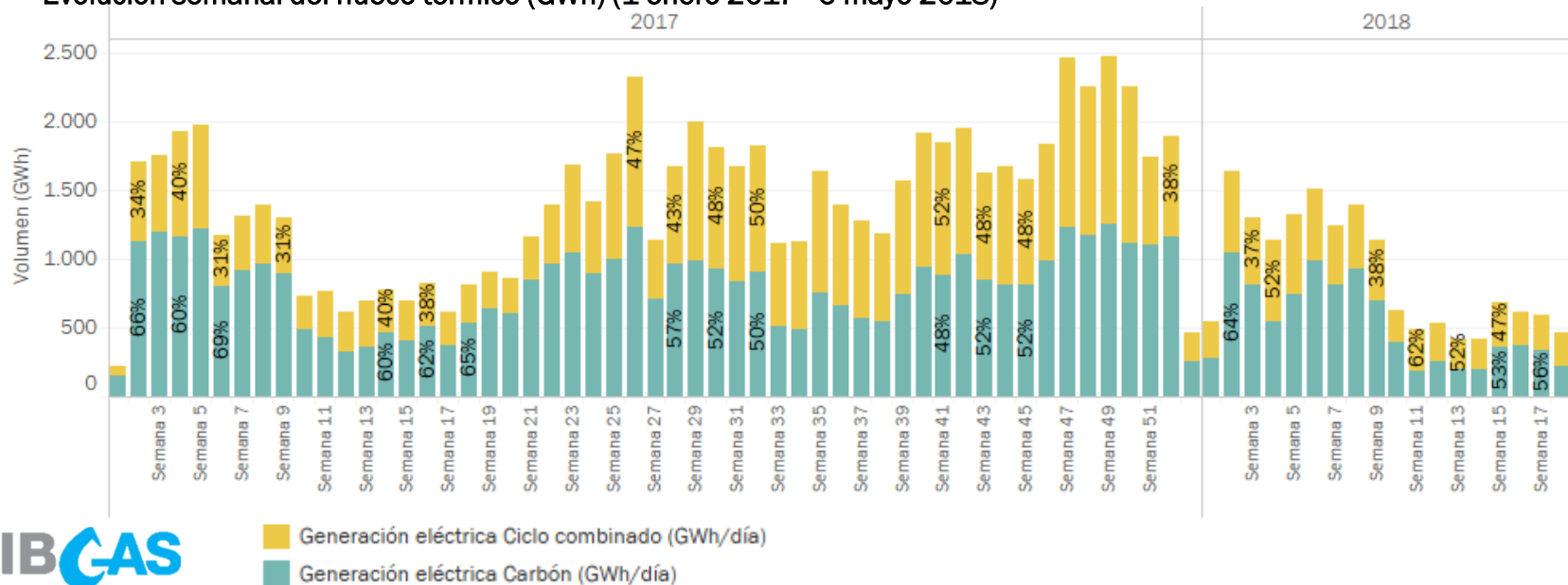
Evolución semanal del hueco térmico (GWh) (1 enero 2017 - 6 mayo 2018)
